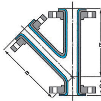
45° Lateral
